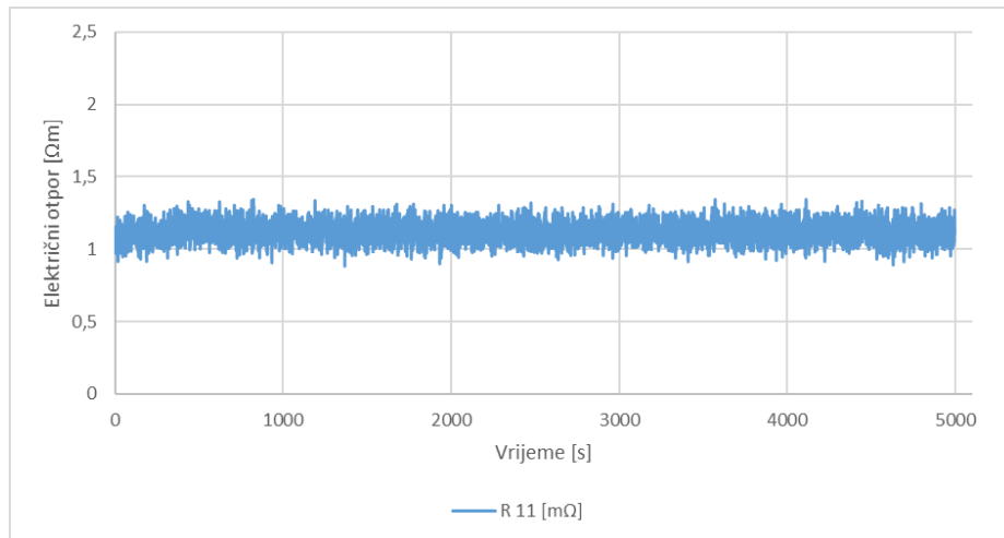
Krivulja promjene električnog otpora – uzorak 11, prevlaka na bazi srebra
