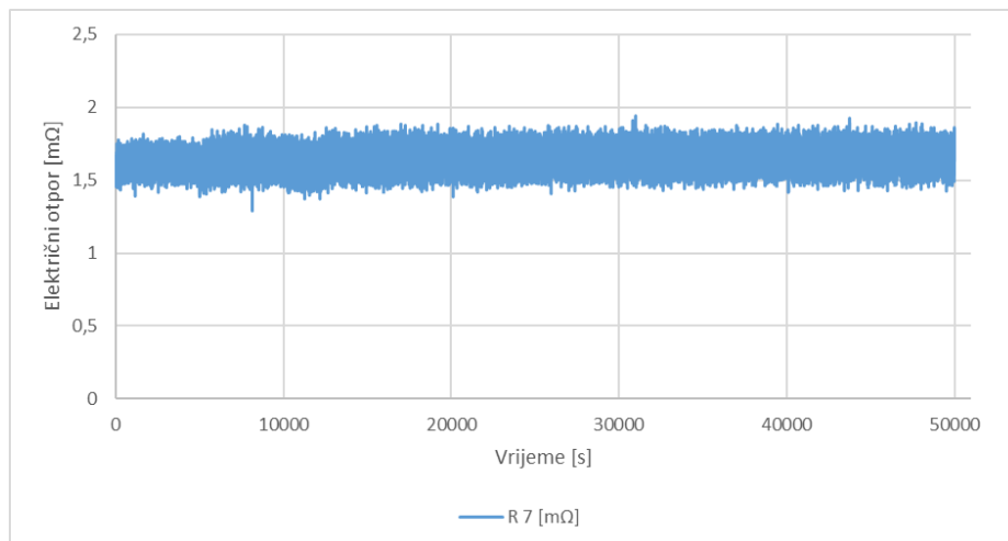
Krivulja promjene električnog otpora – uzorak 7, prevlaka na bazi kositra
