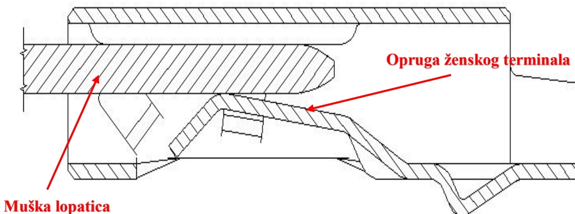
Slika 12. Presjek spoja muškog i ženskog terminala[10]
