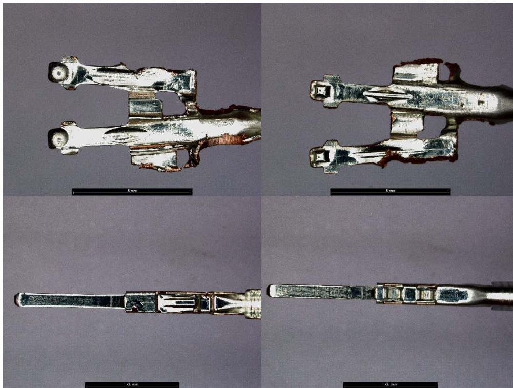
Slika 30 Prikaz muškog i ženskog terminala s kositrenom prevlakom
