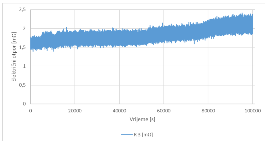
Slika 46. Krivulja promjene električnog otpora – uzorak 3, prevlaka na bazi kositra srebra (ostali dijagrami dani su u Prilogu 1)
