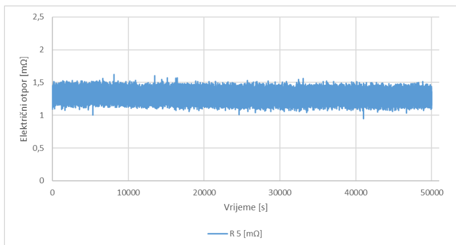
Krivulja promjene električnog otpora – uzorak 5, prevlaka na bazi srebra
