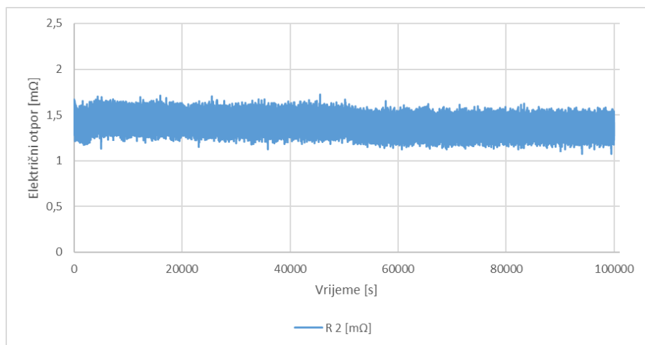
Krivulja promjene električnog otpora – uzorak 4, prevlaka na bazi zlata
