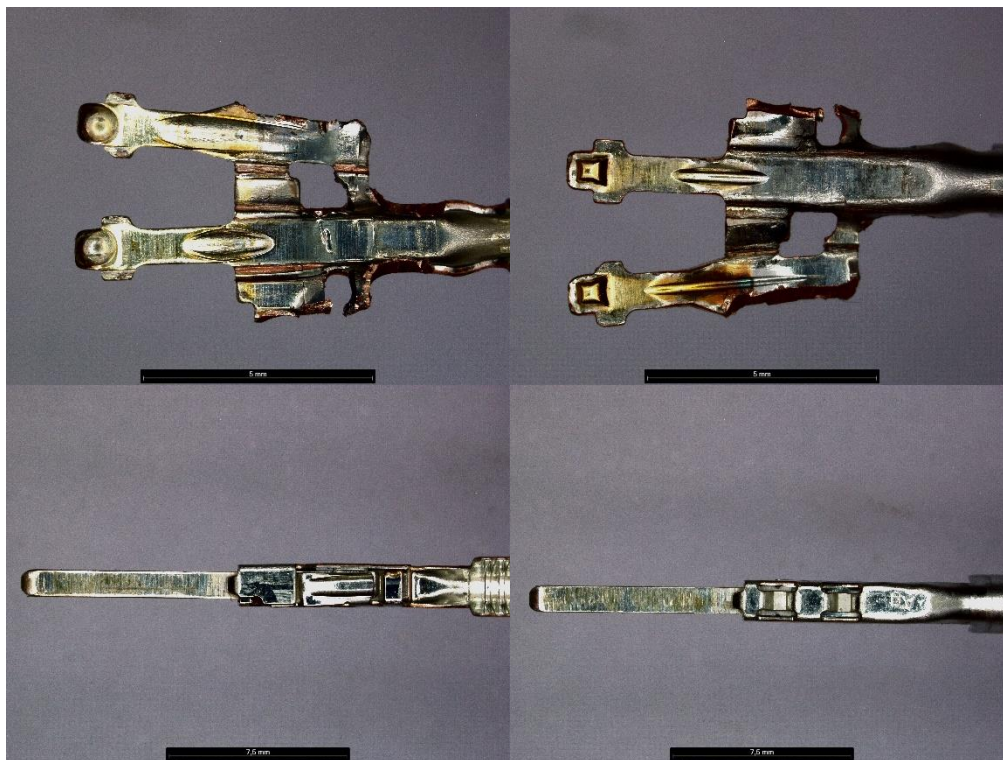
Slika 31 Prikaz muškog i ženskog terminala sa srebrnom prevlakom
