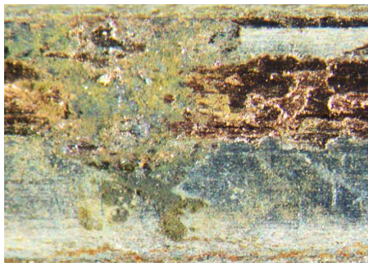
Slika 19. Oštećena kontaktna površina uslijed djelovanja fretting korozije[12]
