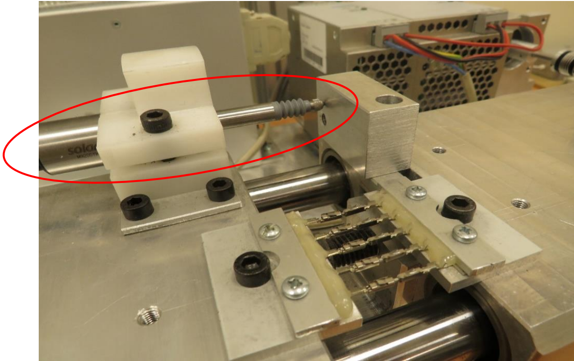
Slika 24. Senzor pomaka
