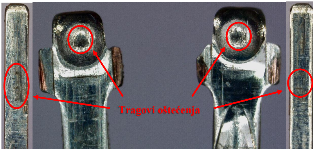
Slika 54. Sn - uzorak 8 nakon 50 000 ciklusa
