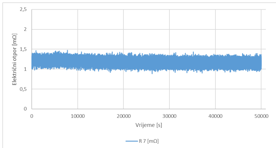
Krivulja promjene električnog otpora – uzorak 7, prevlaka na bazi srebra
