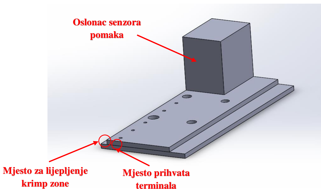
Slika 29. 3D model prihвата terminala na jednoj strani
