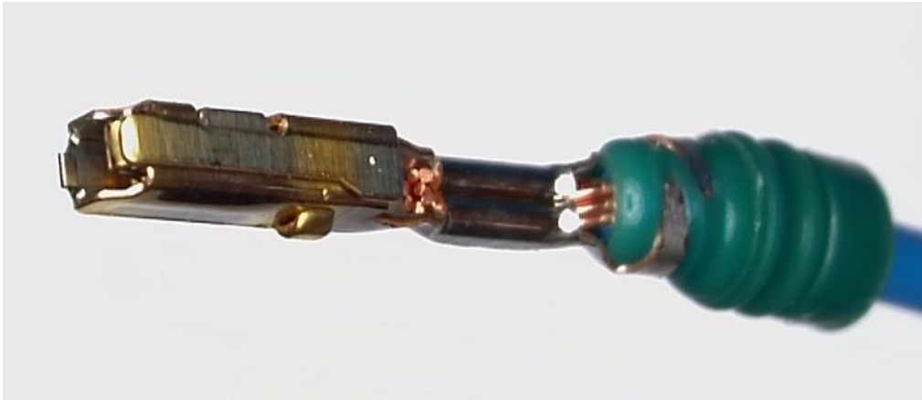
Slika 17. Ženski terminal sa zlatnom prevlakom
