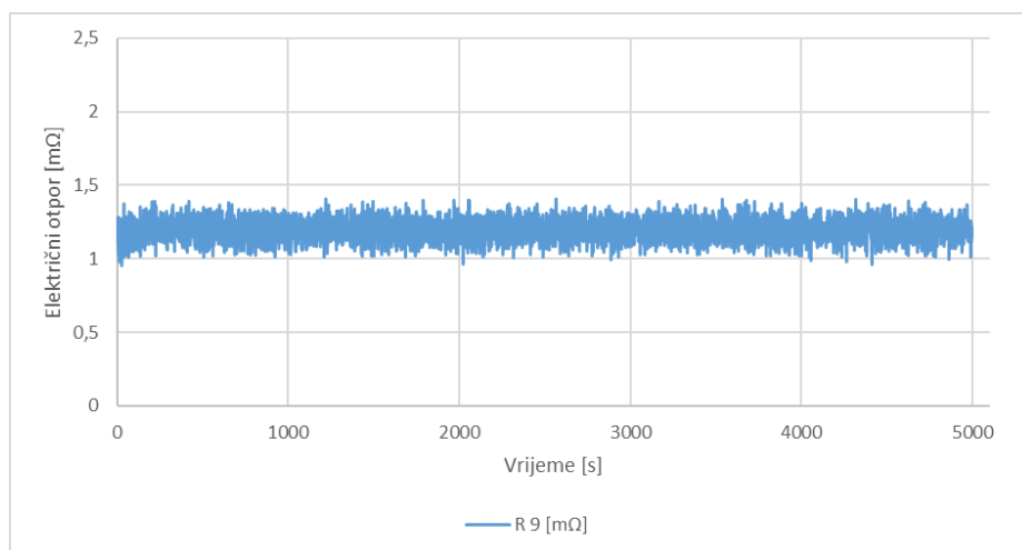
Krivulja promjene električnog otpora – uzorak 9, prevlaka na bazi srebra
