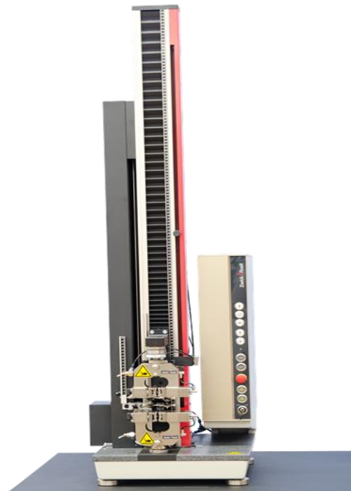
Slika 33. Zwick/Roell Z0.5 [25]
