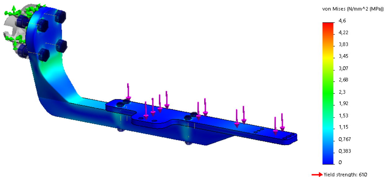
Slika 134. Statička analiza naprezanja modela s korigiranim vrijednostima
