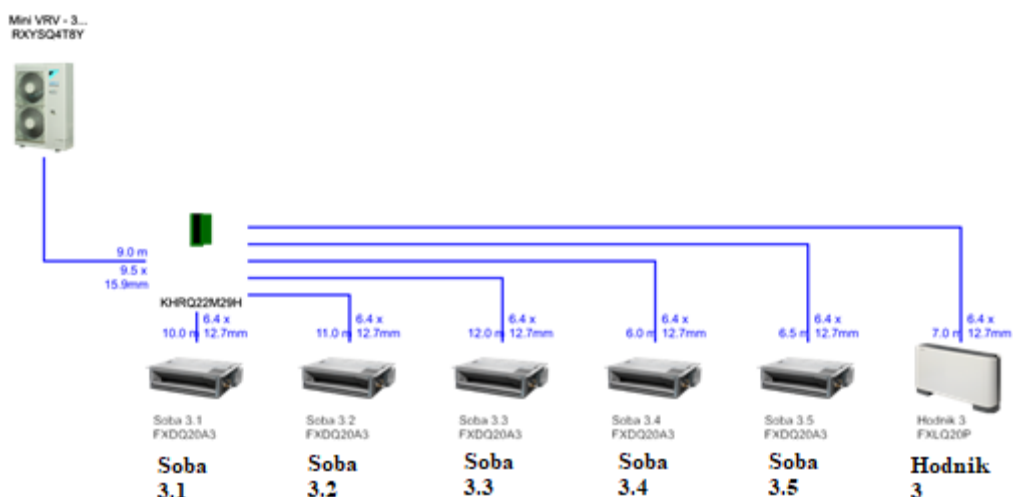
Slika 47. Prikaz izvedbe cjevovoda s češljem - VJ 7 [6]
