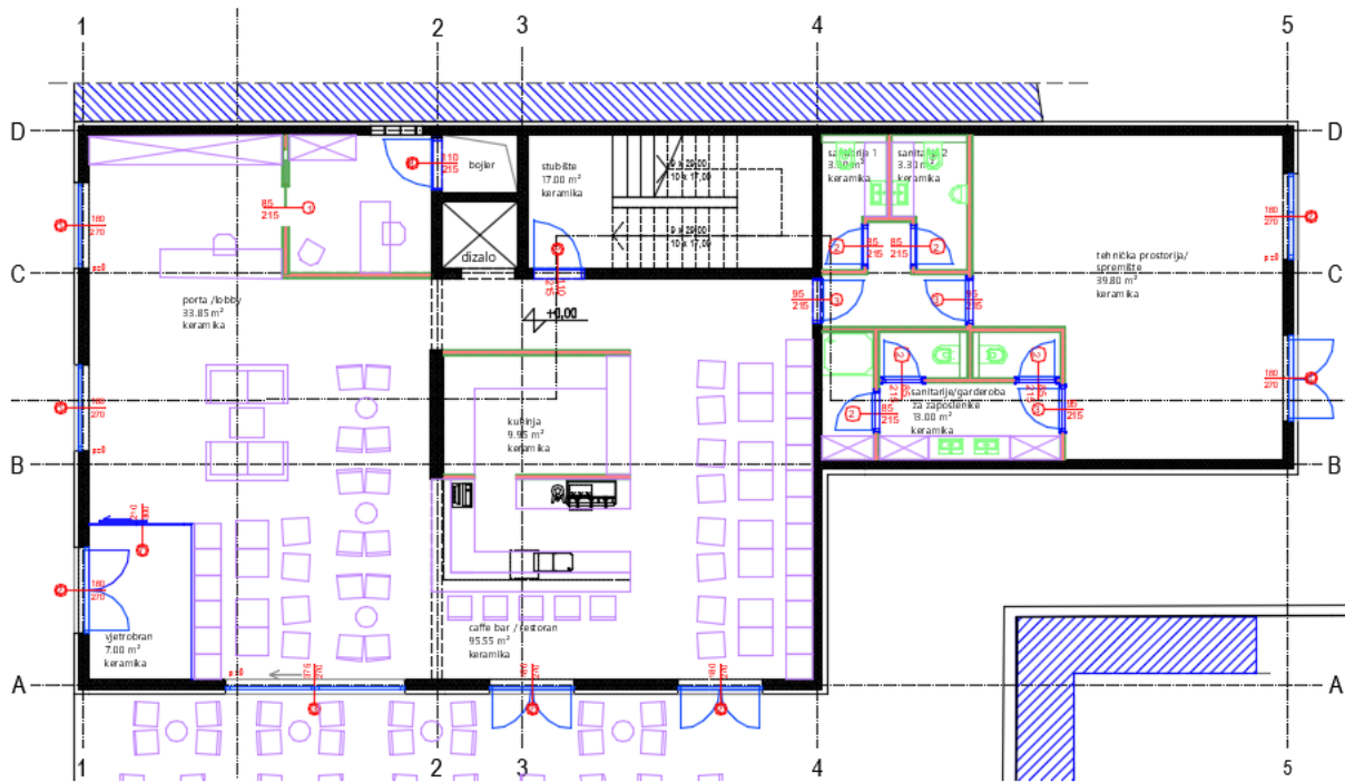
Slika 2. Prizemlje hotela
