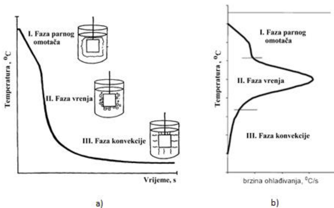
Slika 21. Karakterističan izgled krivulje ohlađivanja (a) ulja za kaljenje i iz nje izračunate krivulje brzine ohlađivanja (b) s označenim fazama ohlađivanja [19]
