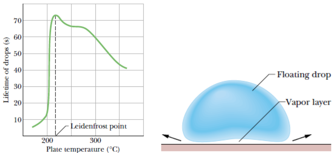
Slika 7. Leidenfrostov fenomen [4].
