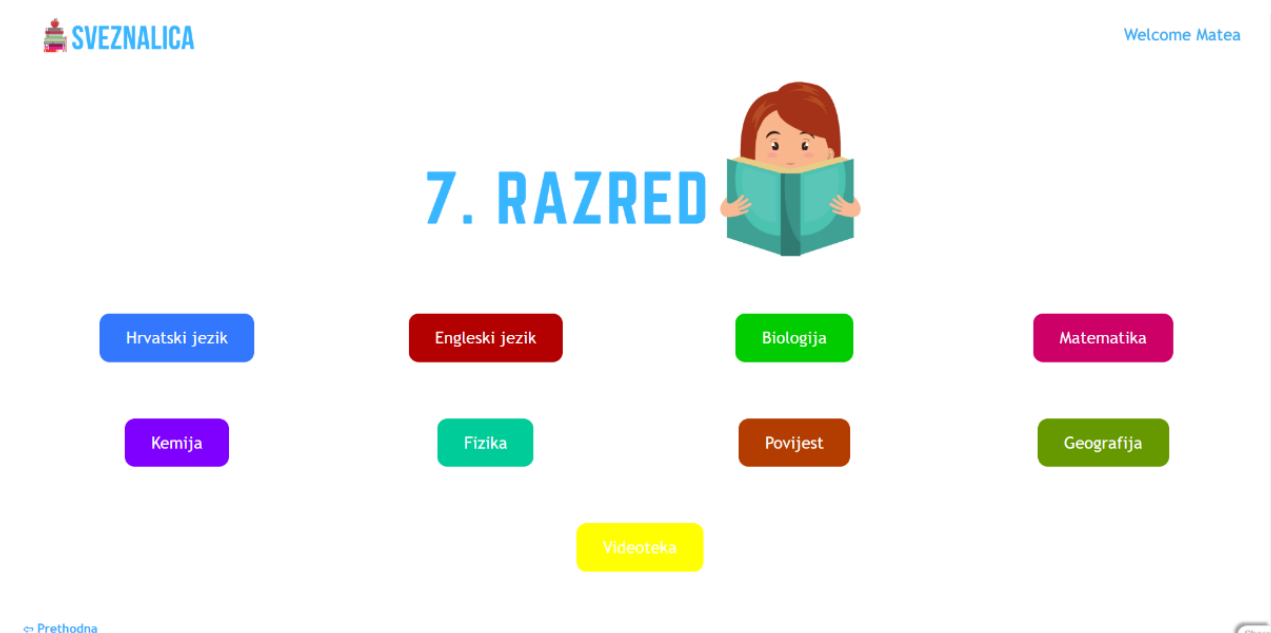
Slika 28. Stranica „7. razred“
