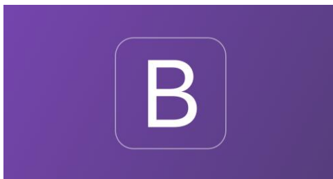
Slika 20. Bootstrap logo
