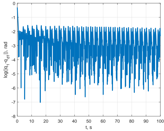
Slika 6.44: Greška praćenja referentne trajektorije q_{d1} u logaritamskom mjerilu za adaptivni regulator uz primjenu neuronskih mreža u horizontalnoj ravnini.
