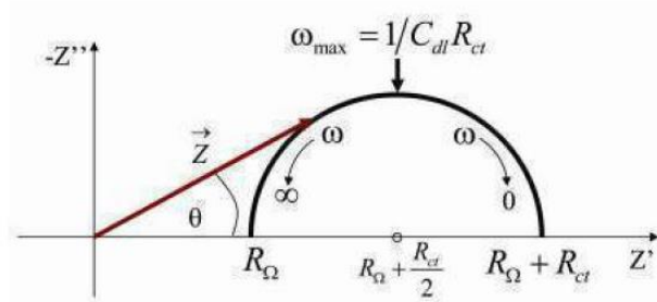
Slika 33. Nyquistov dijagram [10]
