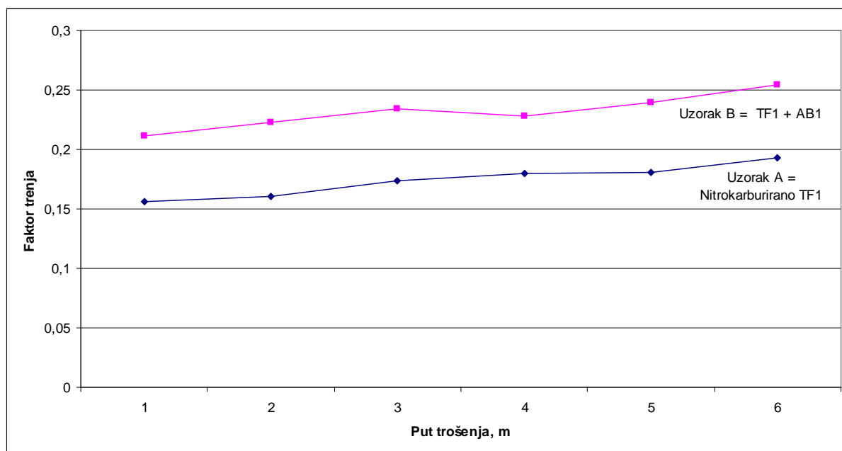
Slika 21. Dijagram ovisnosti faktora trenja o putu trošenja za nitrokarburirani (uzorak A) i nitrokarburirani i naknadno oksidirani ispitni uzorak (uzorak B) (Prilog 3)
