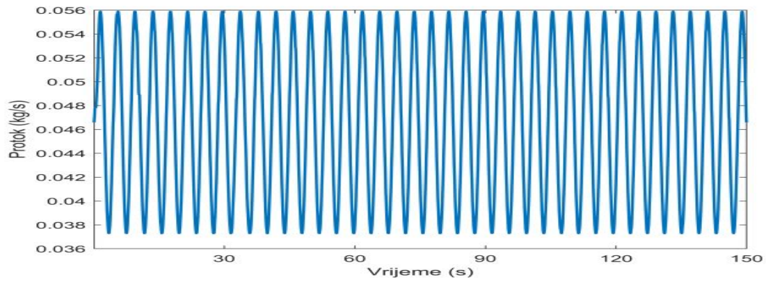
Slika 31. Odstup protoka ogrijevnog medija (ulja) na sinusno opterećenje
