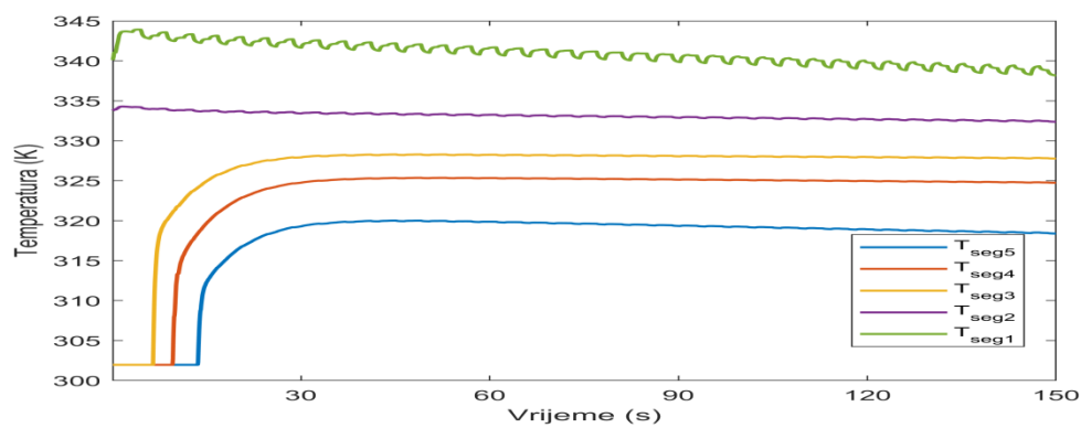
Slika 32. Odstup temperatura segmenata isparivača na sinusno opterećenje
