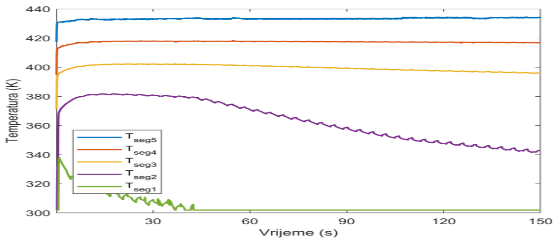
Slika 32. Odstup temperatura segmenata isparivača na sinusno opterećenje
