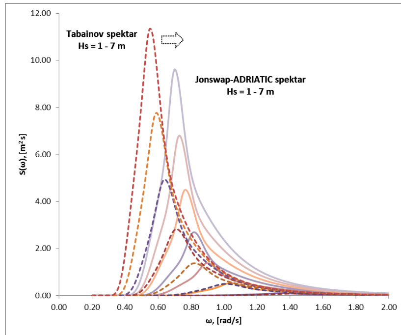
Slika 6-9 Transformacija Tabainovog spektra valova u JONSWAP-Adriatic spektar za unaprijedeni opis valova Jadranskog mora na temelju rezultata numeričkih re-analiza i mjerenja satelitskom altimetrijom
