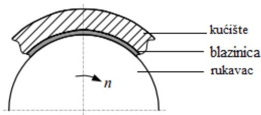
Slika 4. Dijelovi kliznog ležaja [1]
