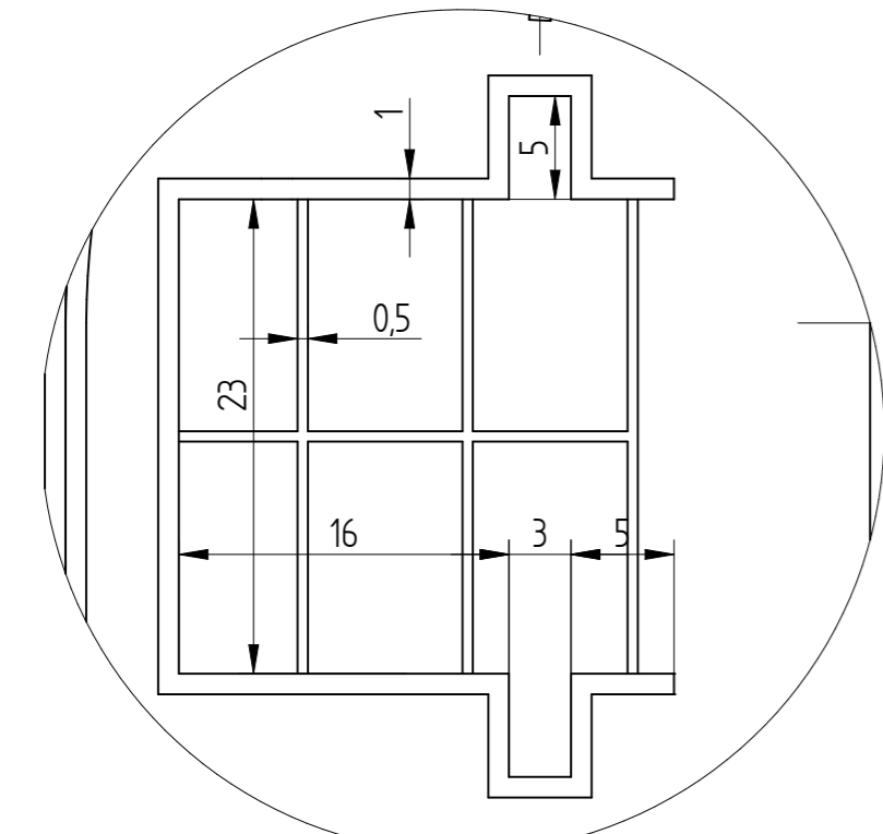
Detalj C M2,5:1
