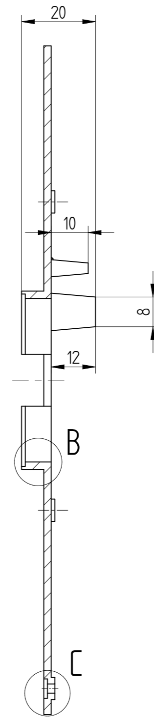
Presjek A-A
