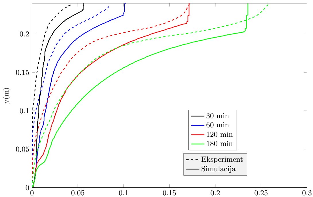
(a) SimE2-L1: C=10^9 , T_s = 306 \text{ }^\circ\text{C} , rjeđa mreža
