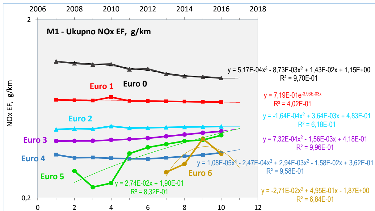
Slika 4.12. Primjer prilagodbe emisijskog faktora vozila flote M1 po emisijskim razinama
