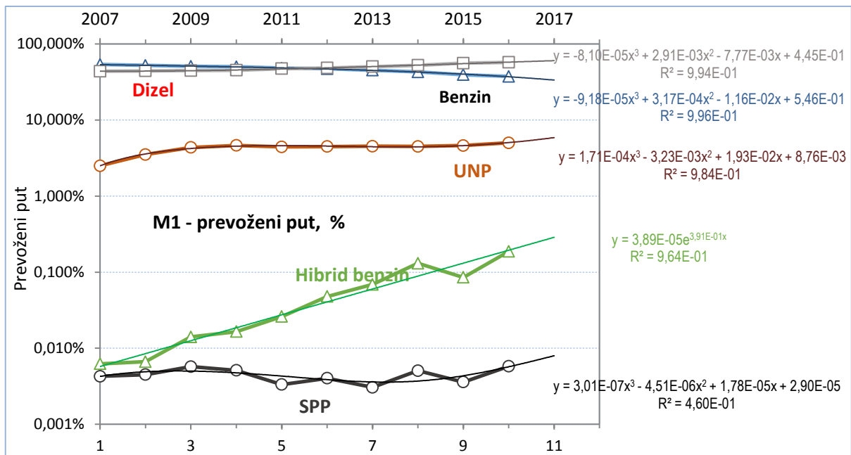
Slika 4.11. Primjer prilagodbe prevoženog puta vozila flote M1 po vrstama pogonskih goriva
