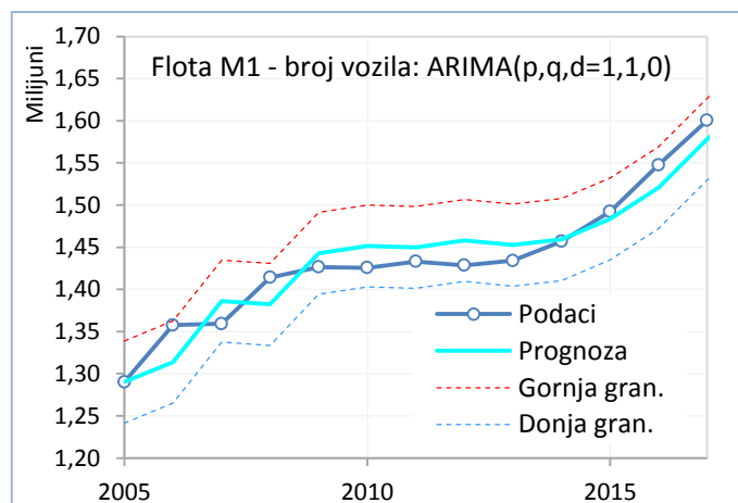
Slika 4.25. Prognostička funkcija forecast modela ARIMA unutar intervala podataka
