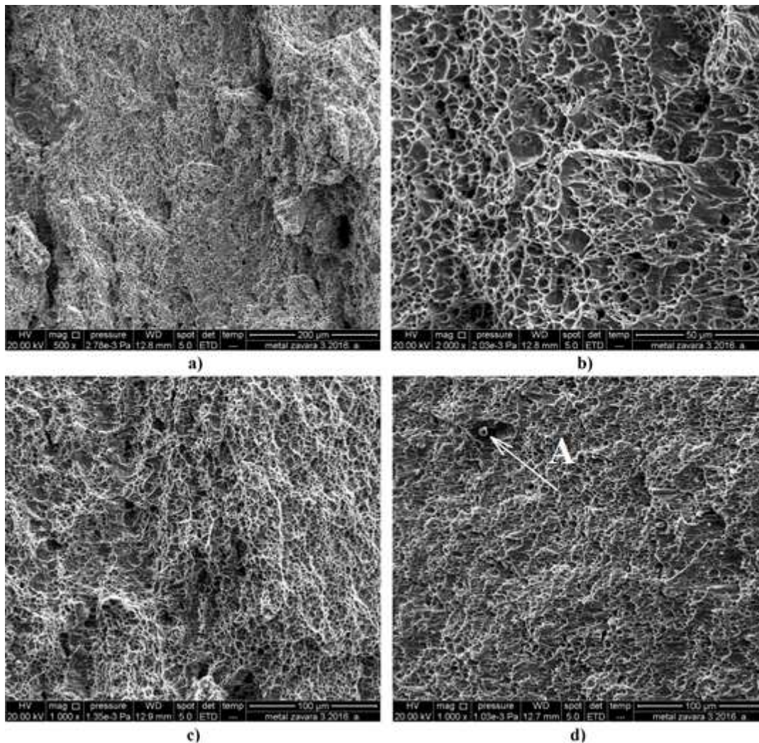
Slika 84. Prijelomne površine MZ, ploča 2D
