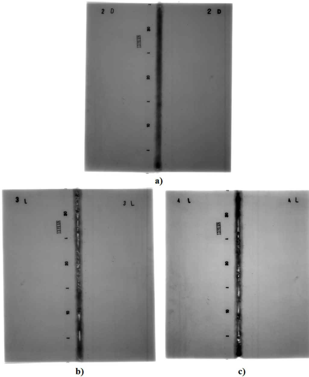
Slika 67. Radiogram ploča:
