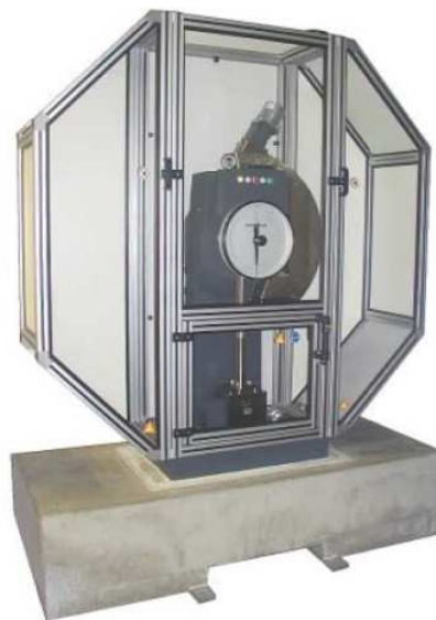
Slika 7. Suvremeni instrumentirani Charpy uređaj [40]
