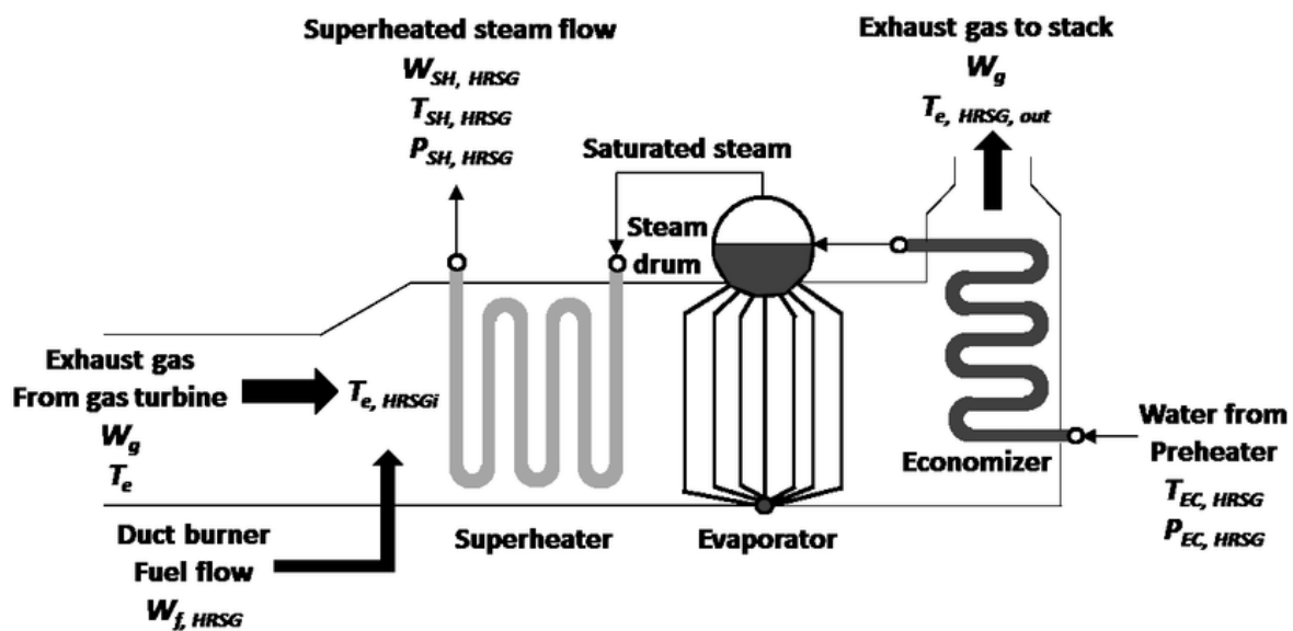
Slika 7. Redoslijed izmjenjivača [7]
