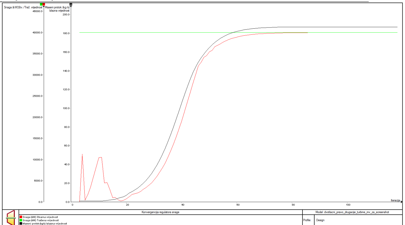
Slika 26. Konvergencija snage generatora s visokim prigušenjem
