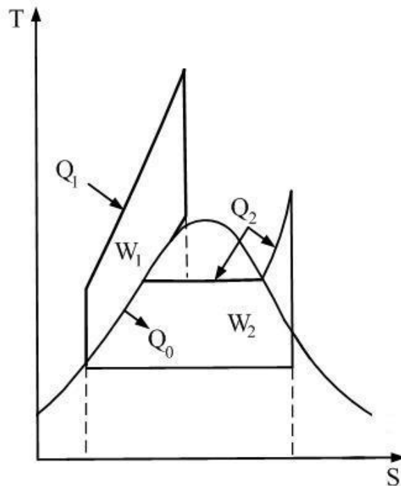
Slika 6. T-s dijagram kombiniranog procesa [6]
