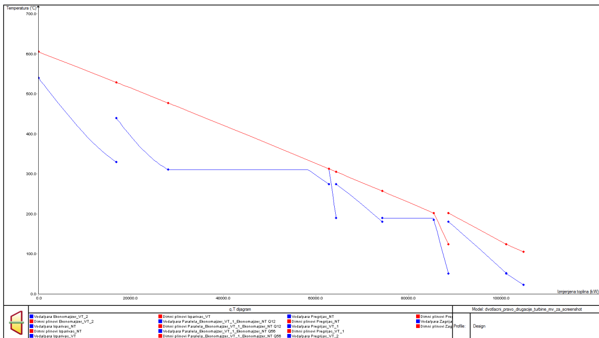
Slika 30. T,Q dijagram procesa
