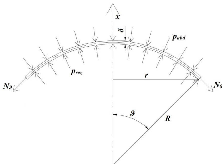
Slika 17. Djelovanje sila i tlakova na puni mjehur
