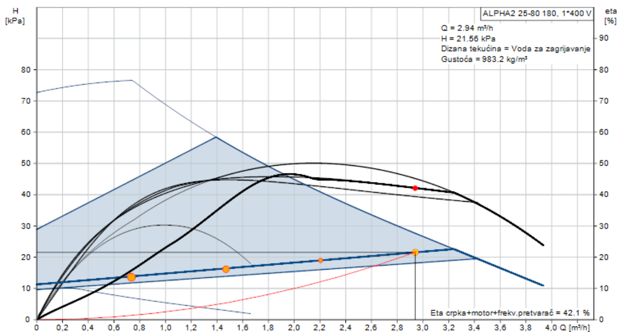
Slika 20. Dijagram radne krivulje pumpe stambenog dijela[13]
