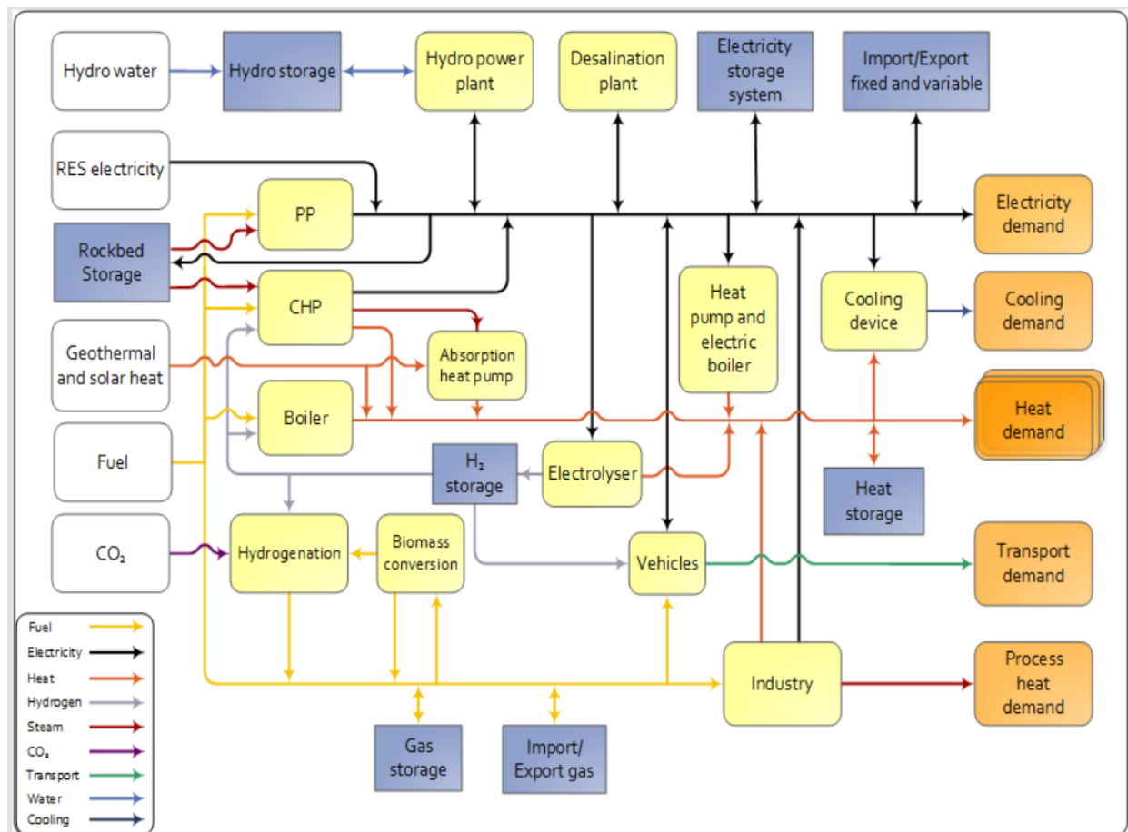
Slika 30: EnergyPLAN shema [47]
