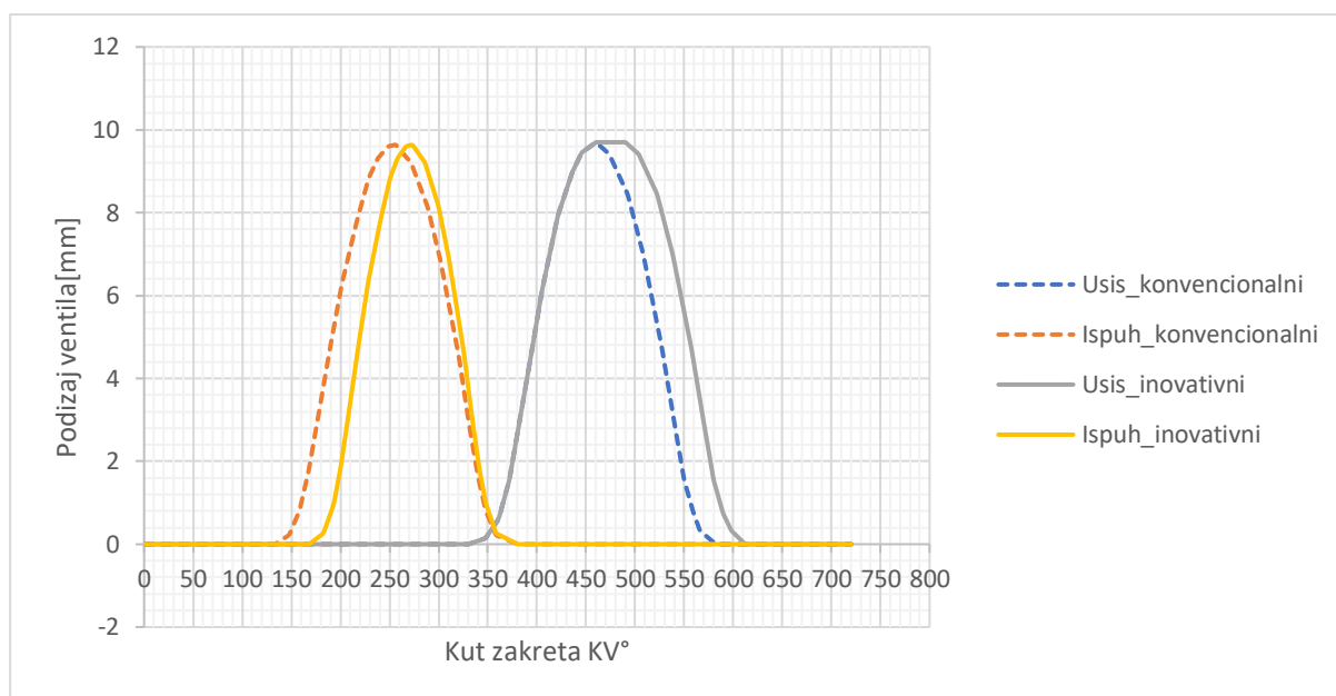
Slika 18. Profil ventila
