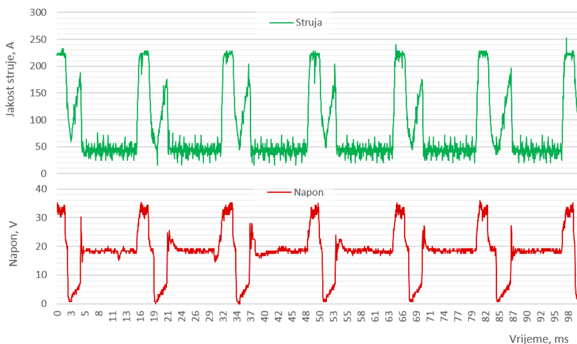
Slika 40. Dinamička karakteristika za prijenos metala impulsnim lukom pri 100 A
