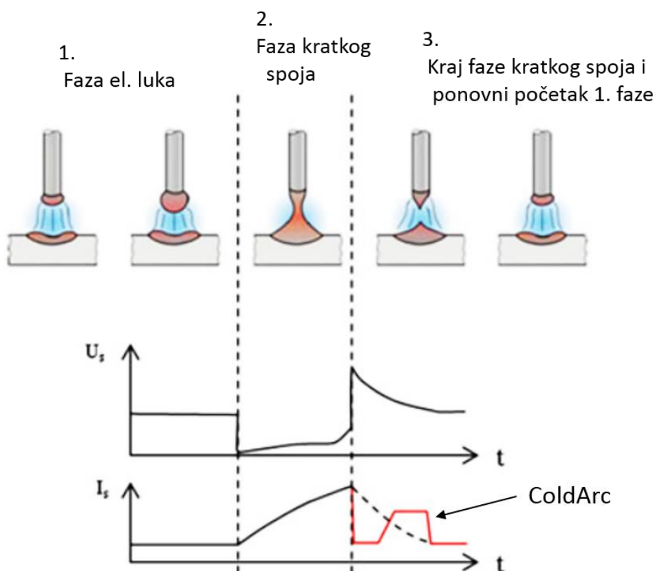
Slika 18. Shematski prikaz principa rada ColdArc postupka [2]
