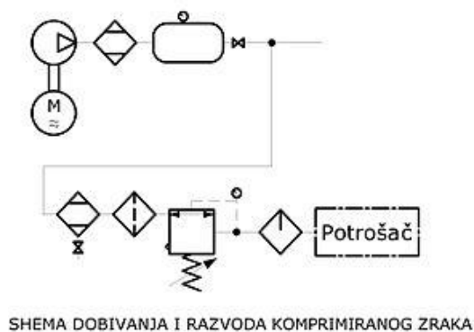
Slika 2. Pneumatski sustav [4]
