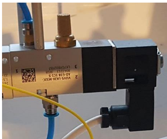
Slika 19. Električki aktivirani 3/2 razvodnik
