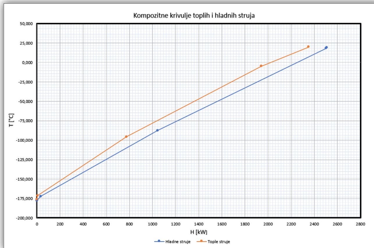
Slika 11: Kompozitne krivulje toplih i hladnih struja
