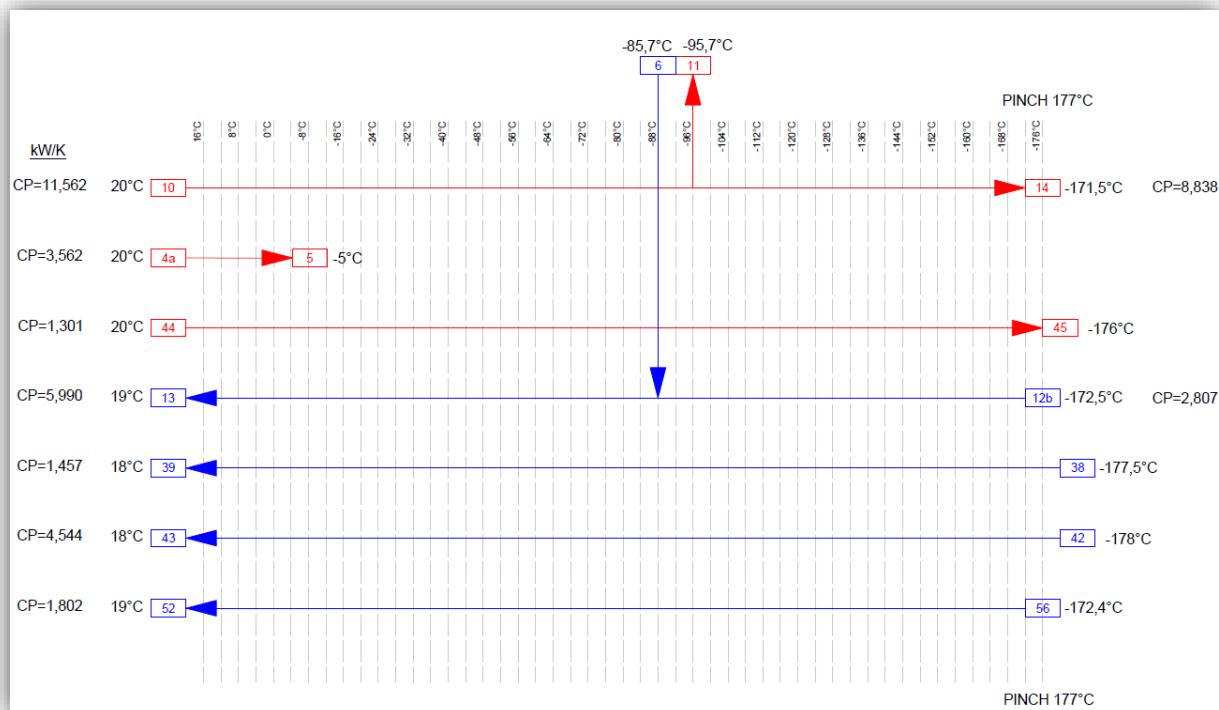
Slika 15: Rešetkasti dijagram struja
