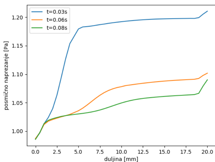
Slika 38. Raspodjela posmičnog napreznaja po duljini vanjske domene za treći slučaj
