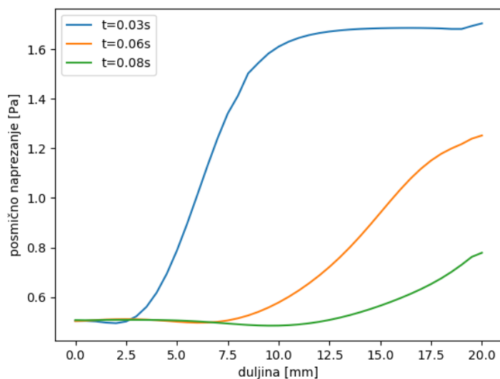
Slika 37. Raspodjela posmičnog napreznaja po duljini unutarnje domene za treći slučaj
