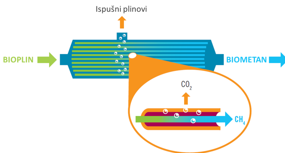
Slika 9.1. Prikaz rada procesa pročišćavanja plina pomoću membrana [17].
