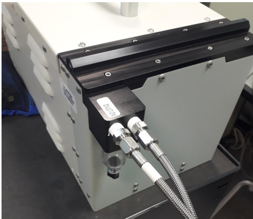
Slika 34. Stražnja strana analizatora s priključenim crijevima za prienos uzorka ispušnih plinova i zraka za razrjeđivanje
