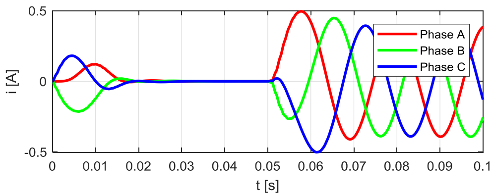
Slika 38. Odziv faznih struja za regulacijski krug brzine vrtnje u A-B-C koordinatnom sustavu
