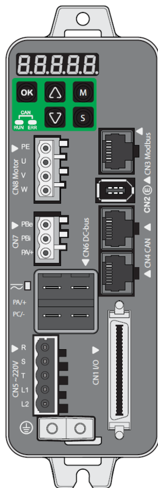
Slika 4. 2D prikaz komponenti i sučelja trofaznog pretvarača snage LXM28A tvrtke Schneider Electric [2]
