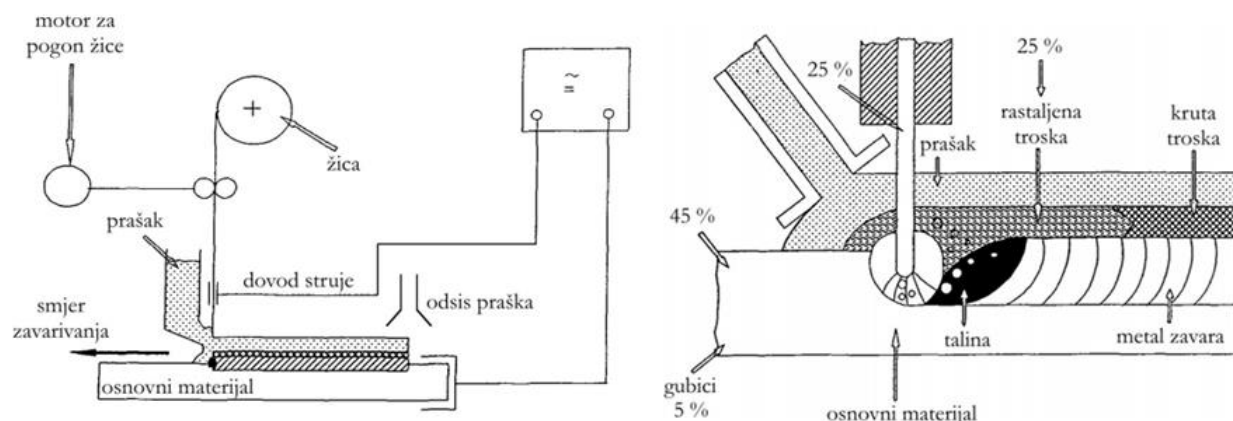
Slika 19. Shema elektrolyučnog zavarivanja pod zaštitom praška (EPP) [19]
