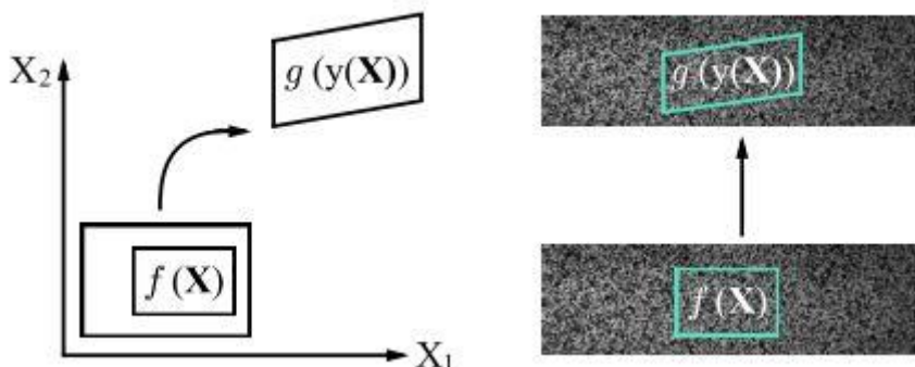
Slika 25. Referenta slika f(\mathbf{X}) deformira se u deformiranu sliku g(\mathbf{y}(\mathbf{X})) [24]
