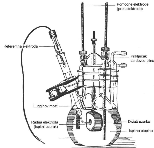
Slika 40. Prikaz elektrokemijske ćelije [17]
