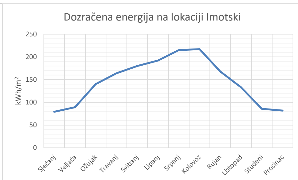
Slika 15. Dijagram dozračene energije na lokaciji Imotski
