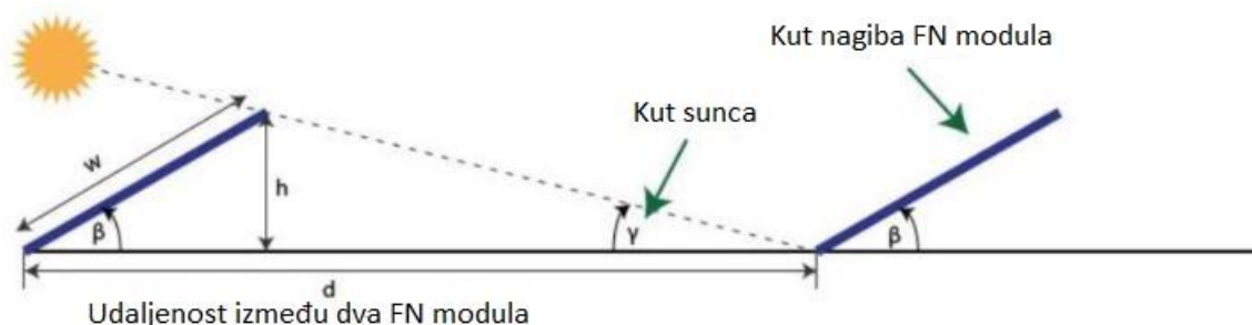
Slika 9. Udaljenost između dva fotonaponska modula
