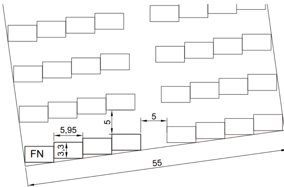
Slika 14. Raspored fotonaponskih modula
