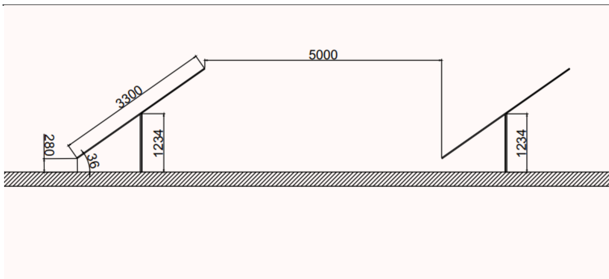
Slika 13. Razmak fotonaponskih modula
