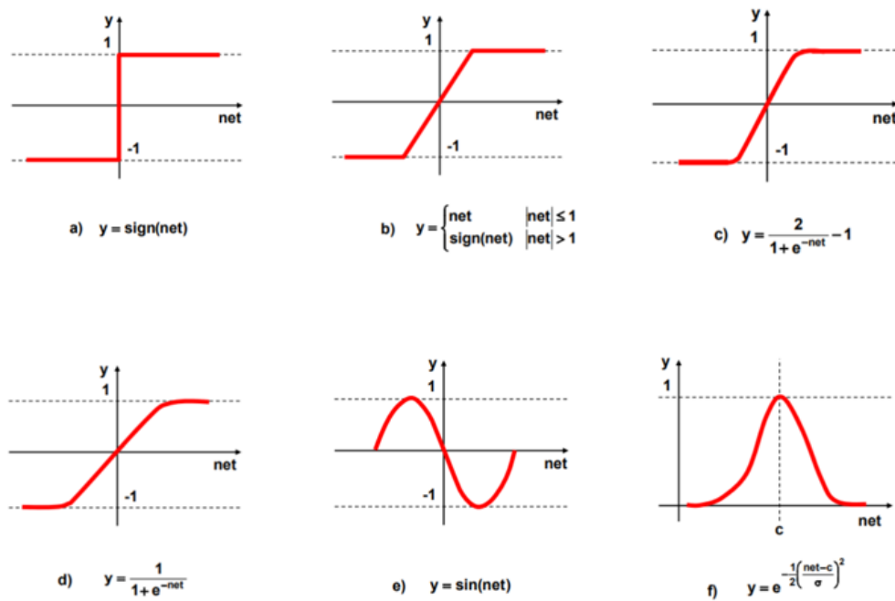
Slika 9. Aktivacije funkcije [13]
