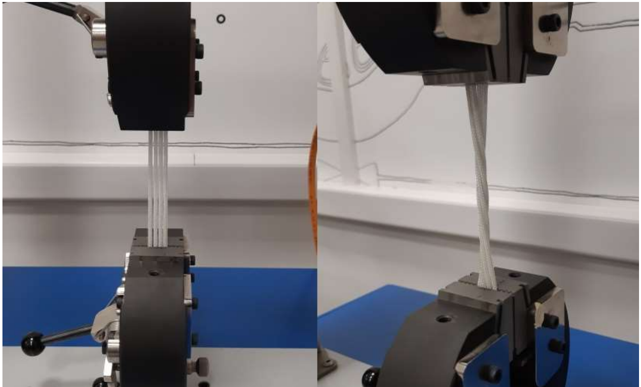
Slika 15. Ispitivanje 4 ravne i 4 uvijene niti užeta
