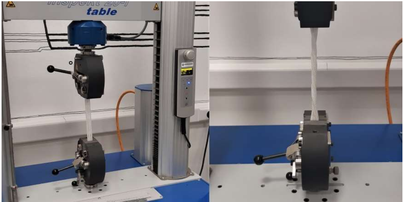
Slika 16. Ispitivanje 3 ravne i 3 uvijene niti užeta
