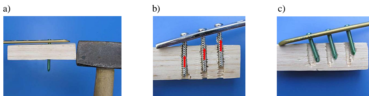
Slika 18. Biomehaničke karakteristike pločice na zaključavanje: a) veća otpornost na smik, b) izvlačenje vijaka kod konvencionalne pločice i c) izvlačenje vijaka kod pločice na zaključavanje [21]
