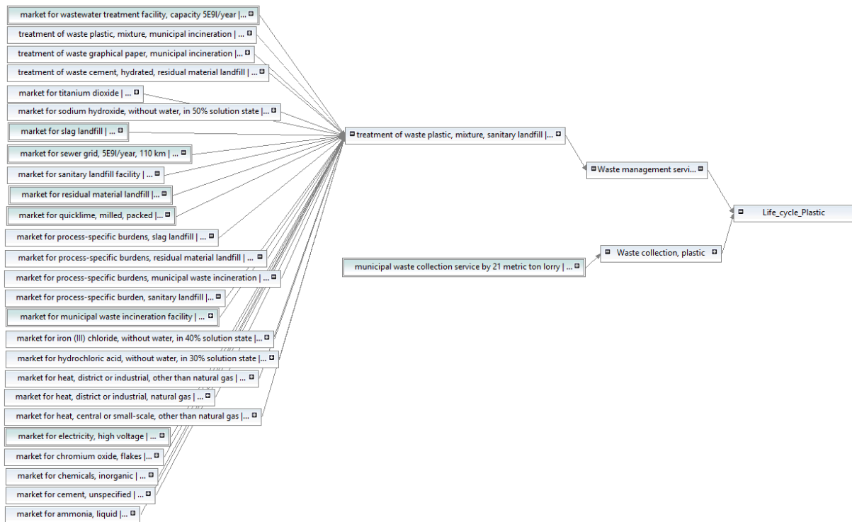
Slika 30. Modeliranje odlaganja
