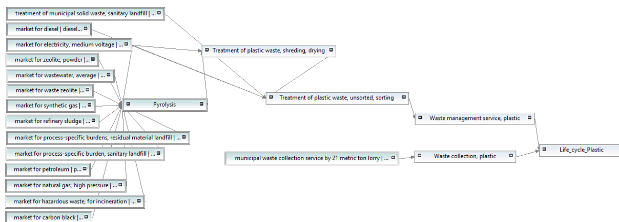
Slika 27. Modeliranje pirolize
