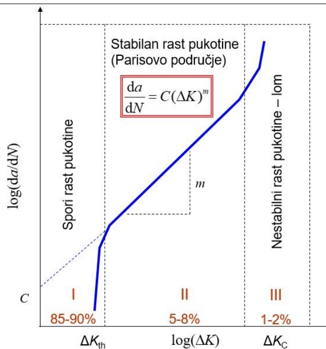
Slika 13. Parisov zakon [8]
