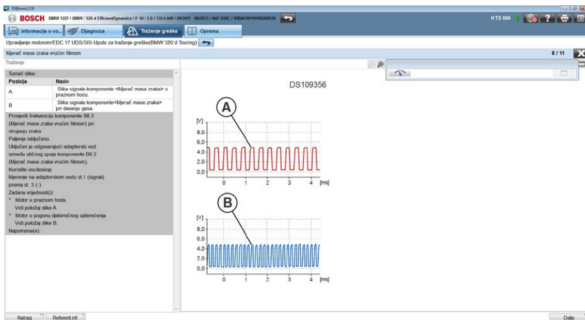
Slika 6.21. Referentni oscilogram mjerača mase zraka vozila BMW 520d prikazan u modulu traženje greške
