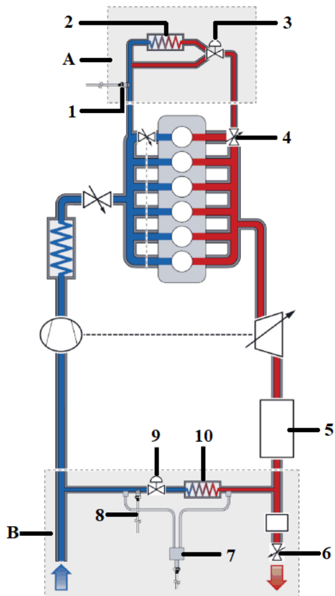
Slika 5.2. Shematski prikaz recirkulacije ispušnih plinova niskog i visokog tlaka [20]
