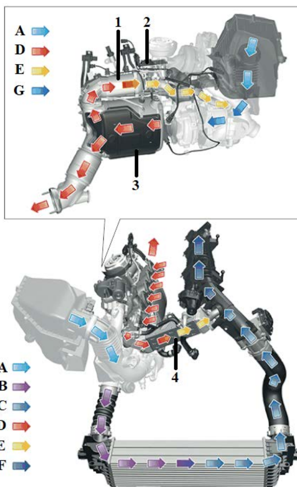
Slika 5.3. Shema strujanja zraka pri recirkulaciji ispušnih plinova visokog i niskog tlaka [20]
