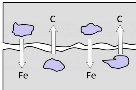
Slika 11. Difuzijsko trošenje [5]
