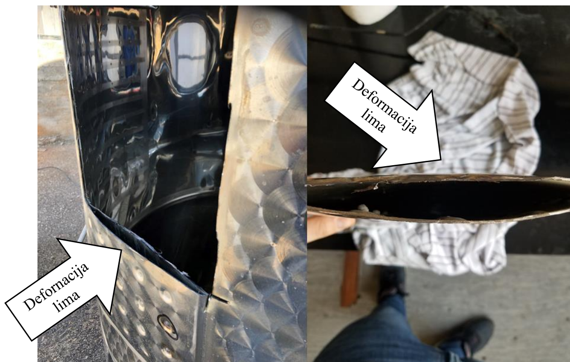
Slika 21. Deformacija lima
