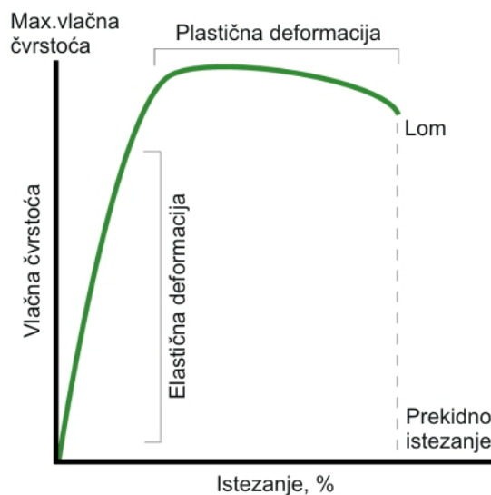
Slika 10 Svojstva materijala [1]
