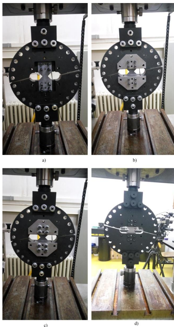
Slika 6.4. Postavljena prirubnica: a) s ispitnim uzorkom, b) s postavljenim tlačnim prihvatom, c) s postavljenim vijcima, podloškama i maticama, d) pogled na prihvatom sa stražnje strane
