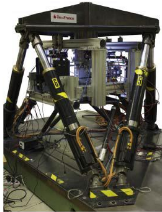
Slika 2.3. 6-osni stroj s odgovarajućim digitalnim kamerama [3]
