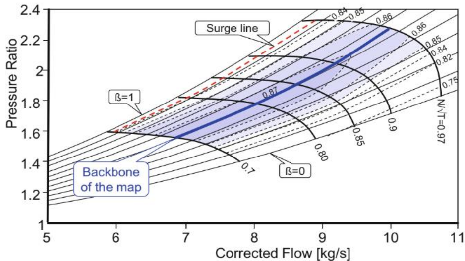
Slika 5: Mapa rada kompresora, [6]
