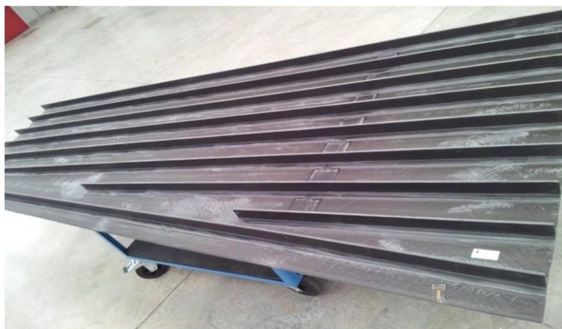
Slika 2. Kompozitni panel krila zrakoplova [1]
