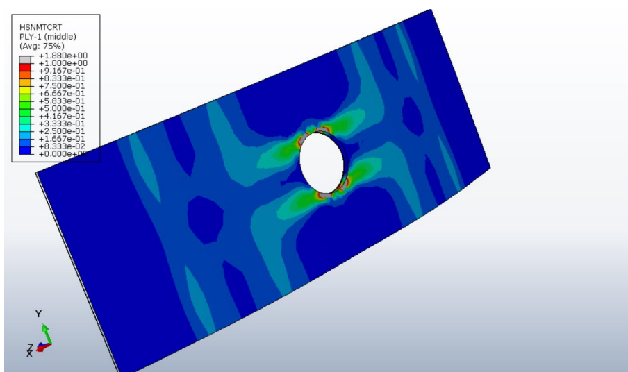
Slika 29. Hashin-ov kriterij za vlačno popuštanje matrice za sloj s postavnim kutom 0^\circ
