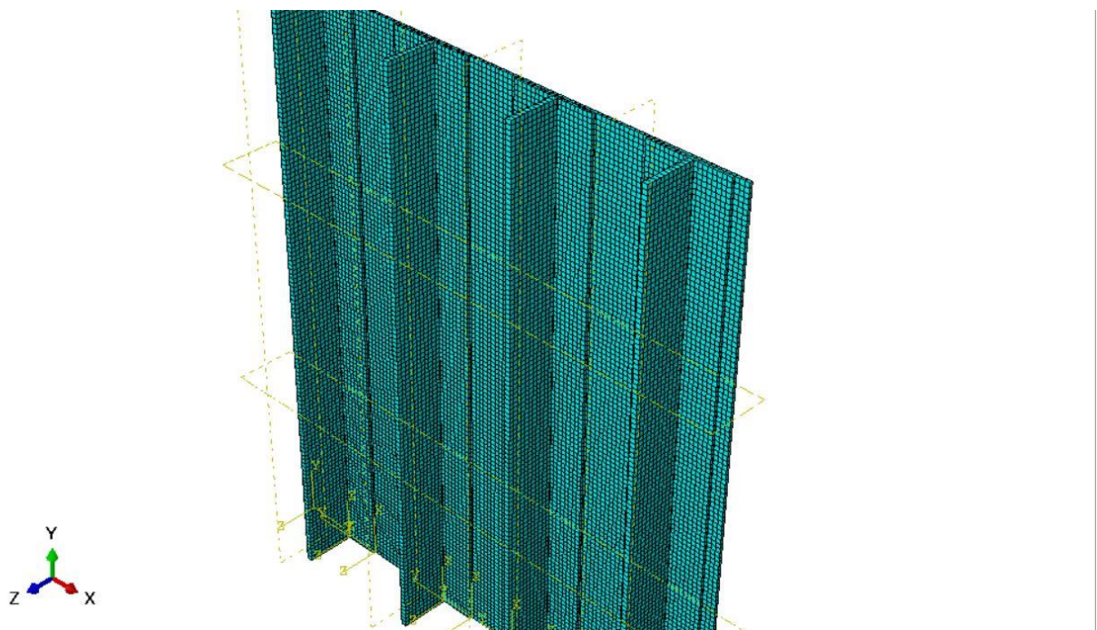
Slika 16. Mreža konačnih elemenata panela ojačanog uzdužnicama
