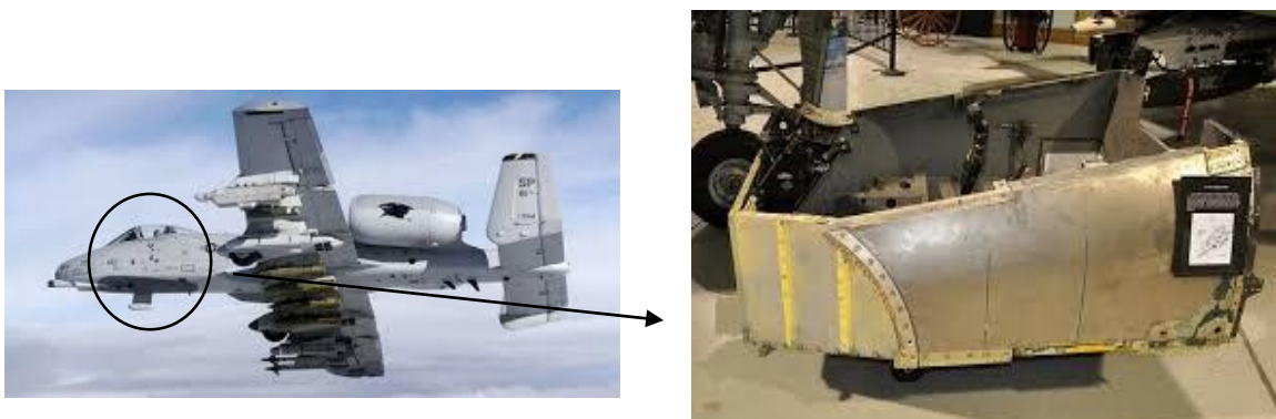
Slika 3. Titanski oklop oko sjedala pilota na zrakoplovu A-10 Thunderbolt II
