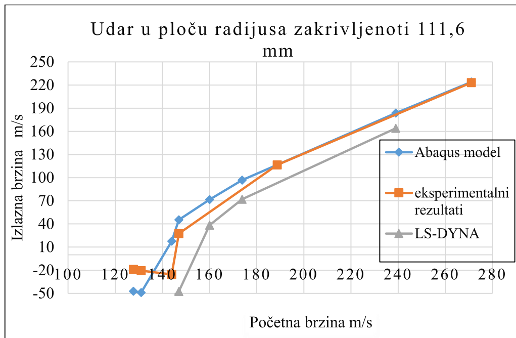
Slika 16. Usporedba rezultata udara u ploču zakrivljenosti 111,6 mm
