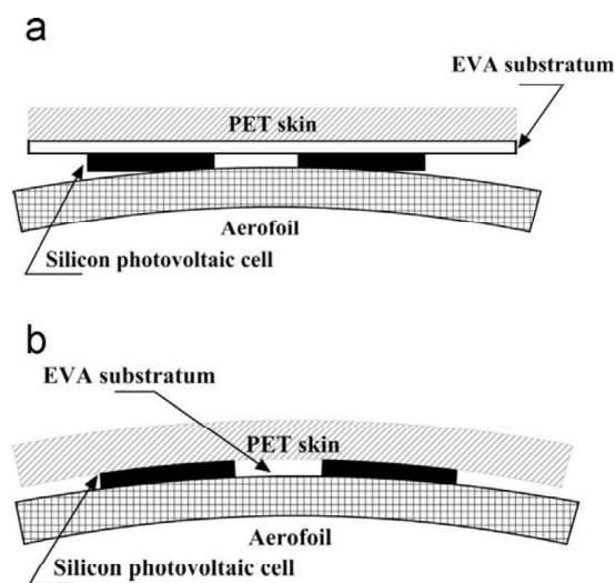
Slika 2.6 Prikaz postavljanja solarnih ćelija na izvoran oblik aeroprofila; a) kruće solarne ćelije b) fleksibilnije solarne ćelije [9]
