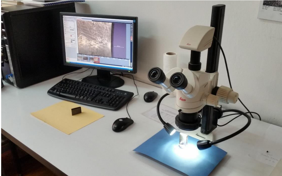
Slika 24: Stereomikroskop Leica MZ6 – Laboratorij za zaštitu materijala FSB-a.
