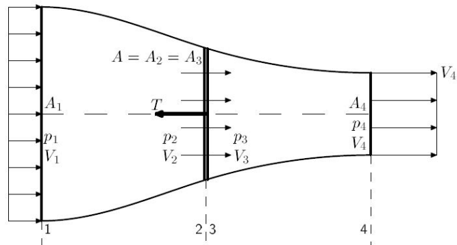
Slika 2.1: Strujna cijev kroz disk propelera [1]
