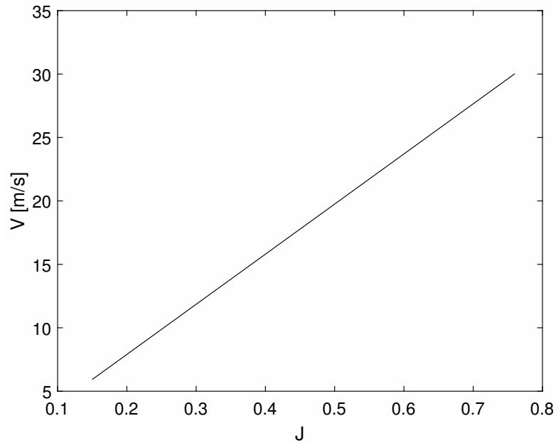
Slika 4.9: Pripadajuće brzine za raspon koeficijenata napredovanja
