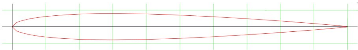
Slika 3.6: Aeroprofil NACA0008 [22]
