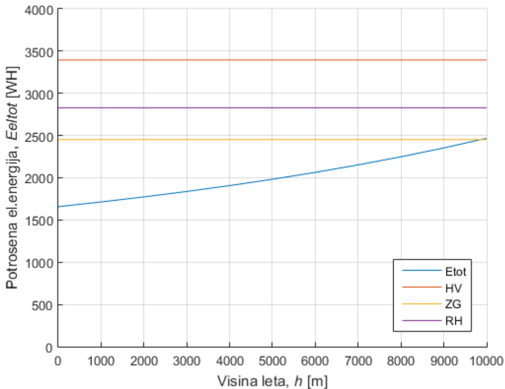
Slika 3.10: Ovisnost potrošene električne energije o visini leta
