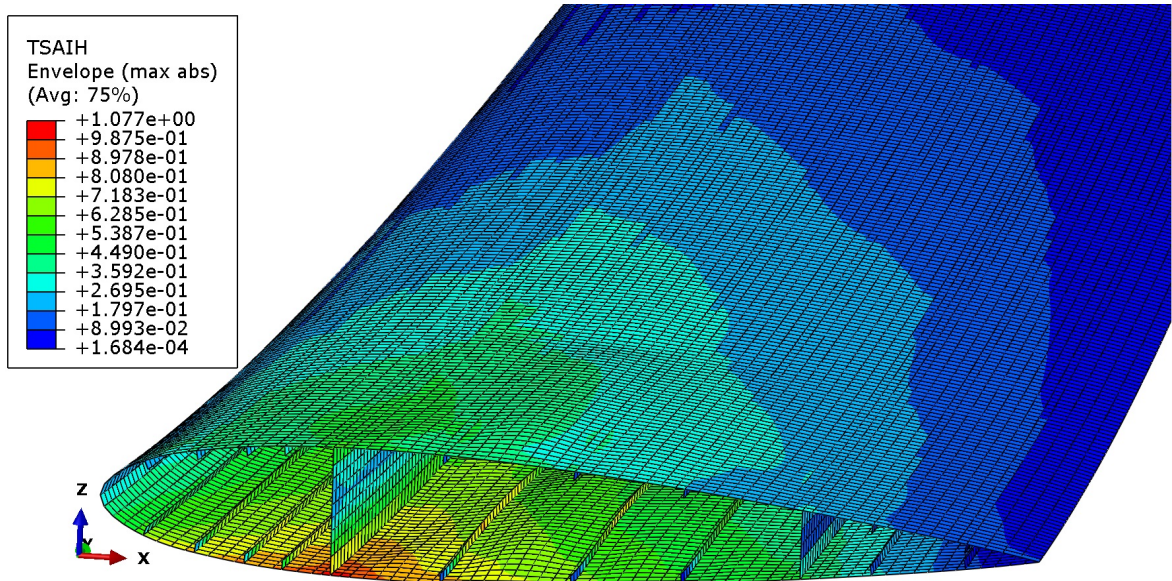
Slika 6.17: Popuštanje kompozita prema Tsai-Hill kriteriju
