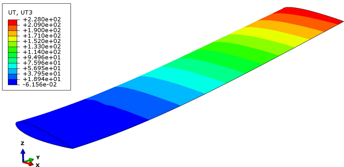
Slika 6.6: Raspodjela pomaka u smjeru globalne osi z uz faktor povećanja 4 za točku C [mm]
